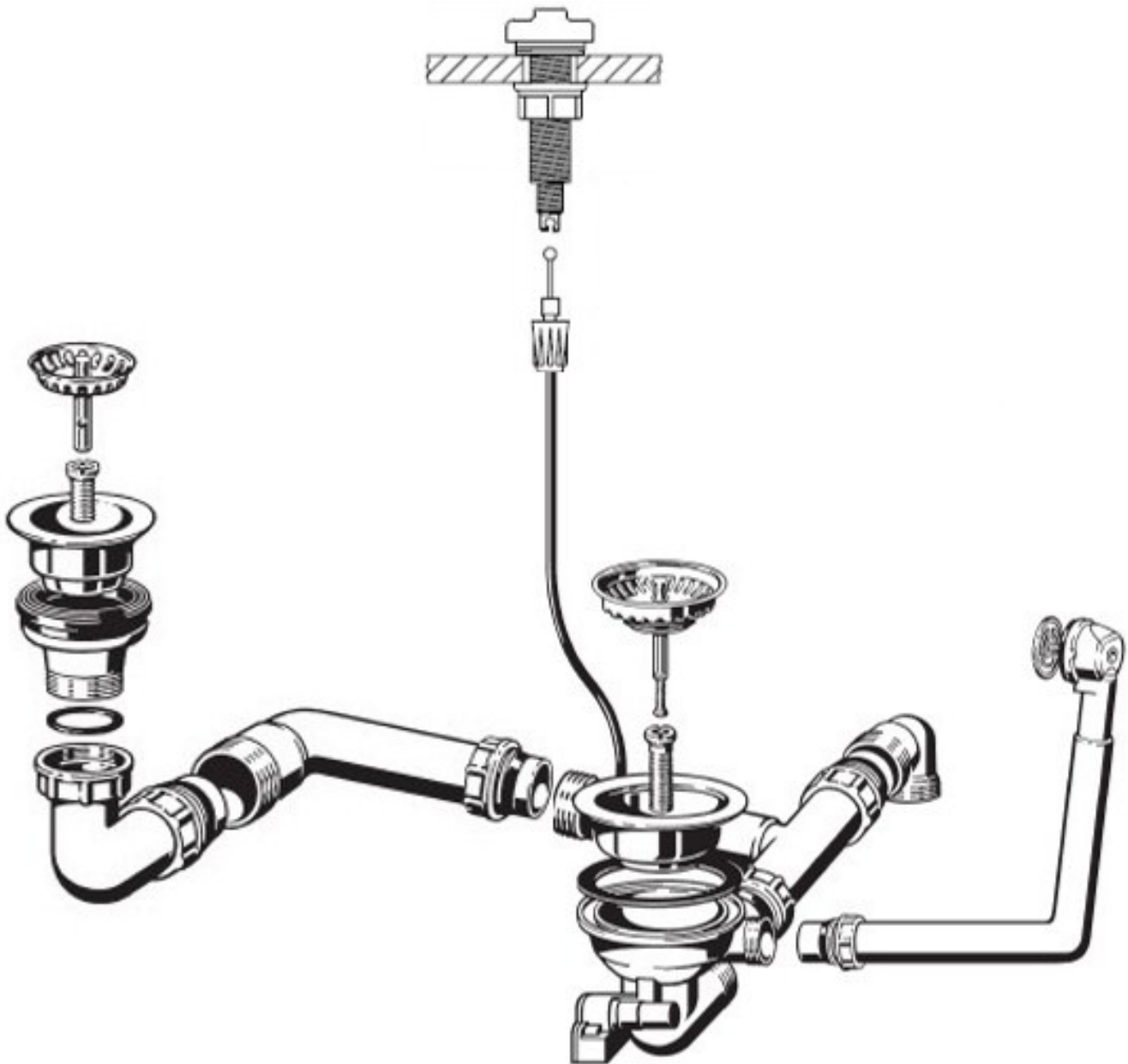
Ablaufgarnitur mit Excenterbetätigung 1 x 3 1/2" + 1 x 1 1/2"
